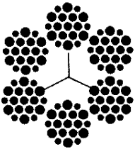
Warrington 6x19 hasta diámetro 5/16"
