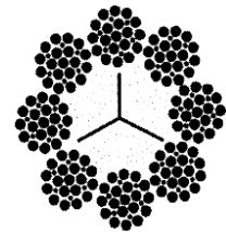
Alambre de relleno 8 x 25 diámetro 1/2" y mayor
