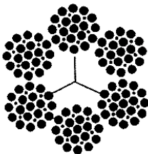
Alambre de relleno 6x25 diámetro 3/8" y mayor
