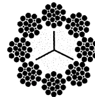
Alambre de relleno 8 x 25 diámetro 1/2" y mayor
