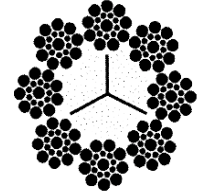
Alambre de relleno 8 x 21 diámetro 1/2" y mayor
