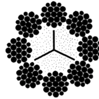
Warrington 8 x 19 hasta diámetro 7/16"
